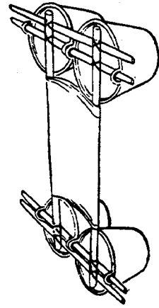
图 3-117 行军锅浮筏
