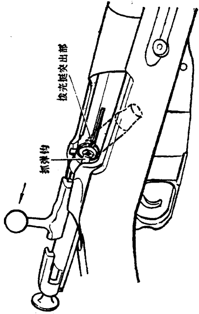
图 2-13 退壳
