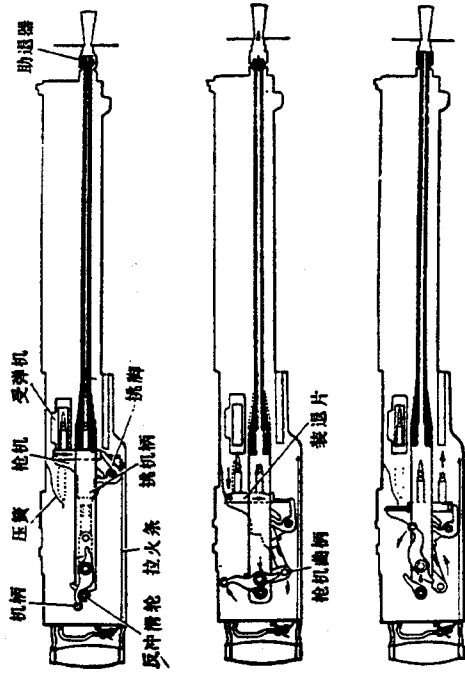
图 2-70 闭锁、开锁和复进
