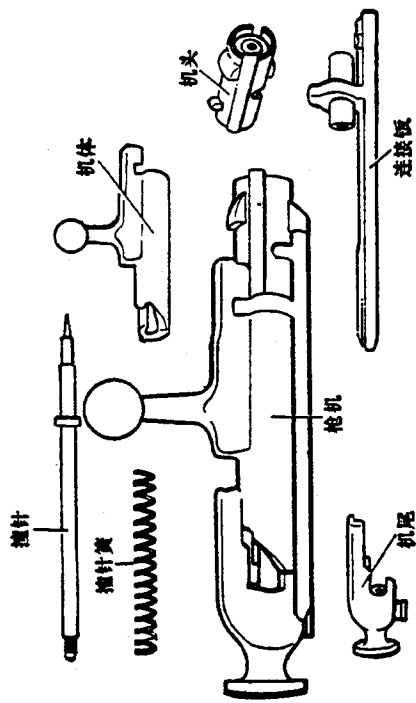
图 2-9 枪机
