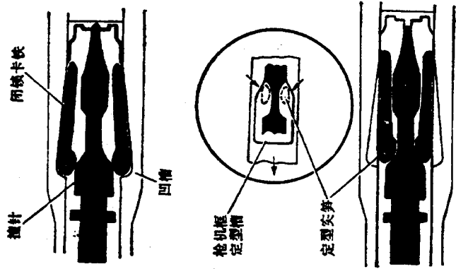
图 2-47 闭锁与开锁
