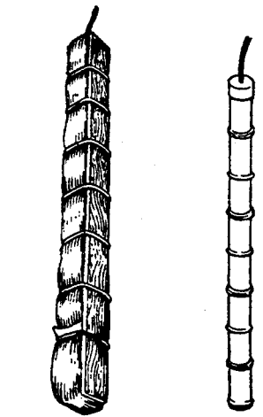
图 3-56 直列装药
