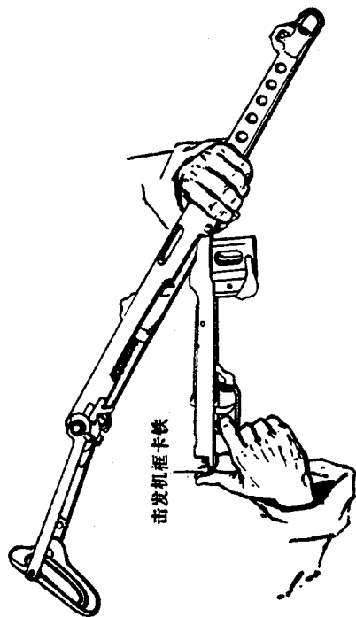
图 2-39 打开机匣
