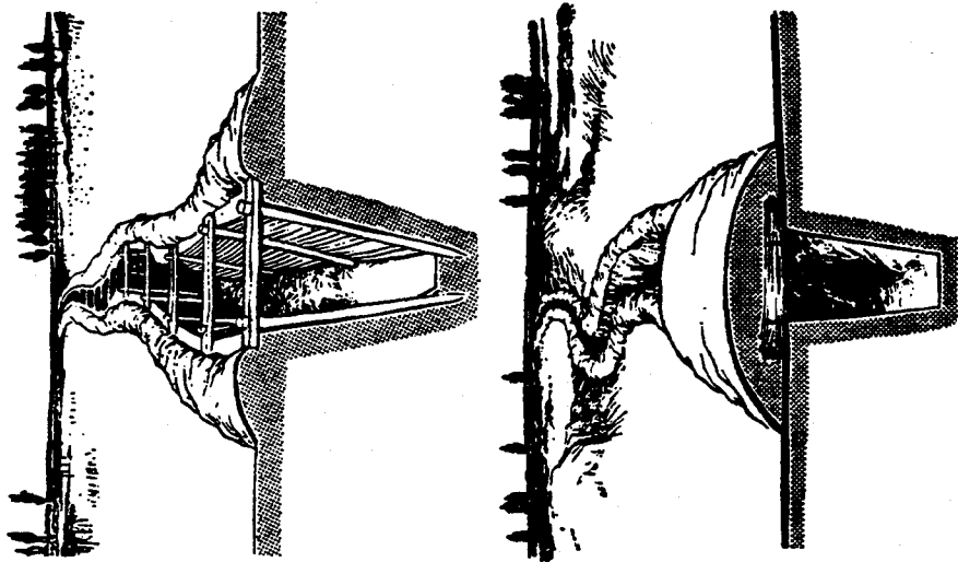
图 7-6 用就便材料被覆加固
