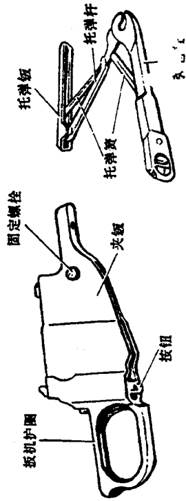
图 2-14 弹仓
