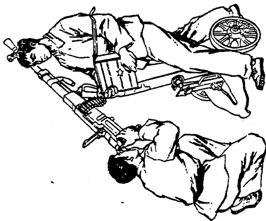
图 2-83 高射架枪
