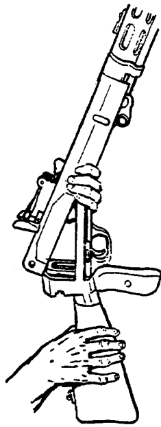
图 2-55 卸下击发机框和木托
