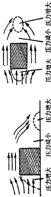
图 7-20 地形地物对冲击波的防护原理
