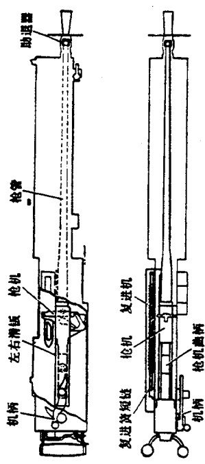
图 2-65 构造示意图
