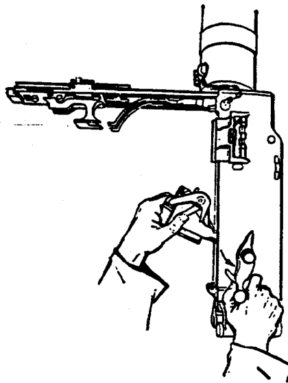
图 2-75 取出枪机
