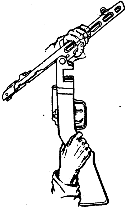
图 2-36 打开机匣
