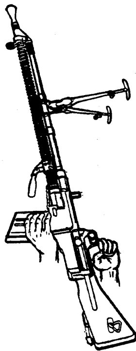
图 2-61 卸下弹匣
