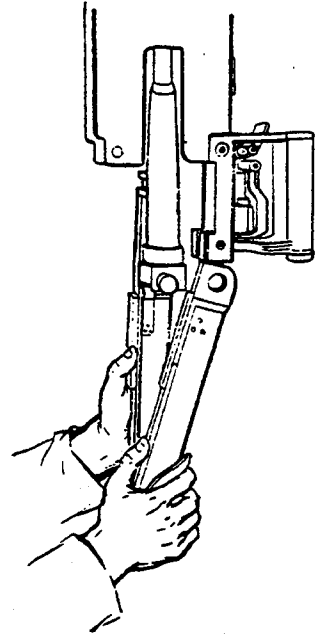
图 2-78 取出左右滑板和枪管
