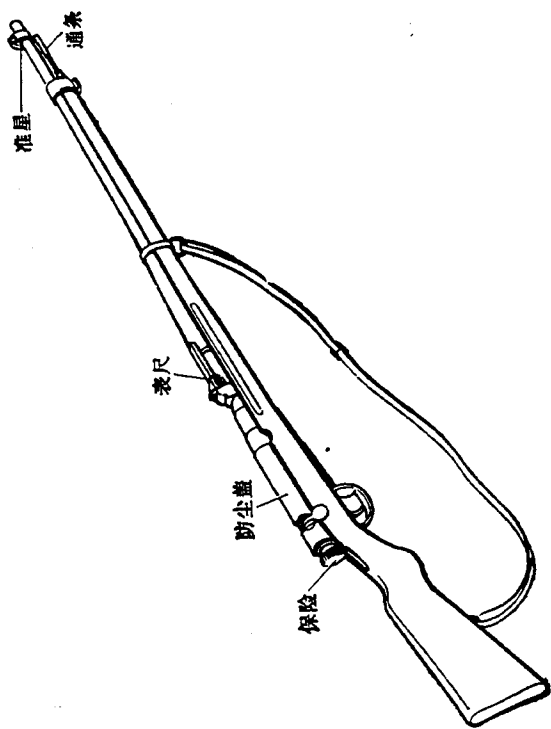
图 2-27 六五步枪
