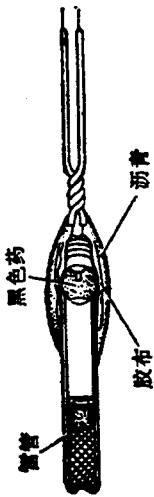
图 3-61 自制电雷管
