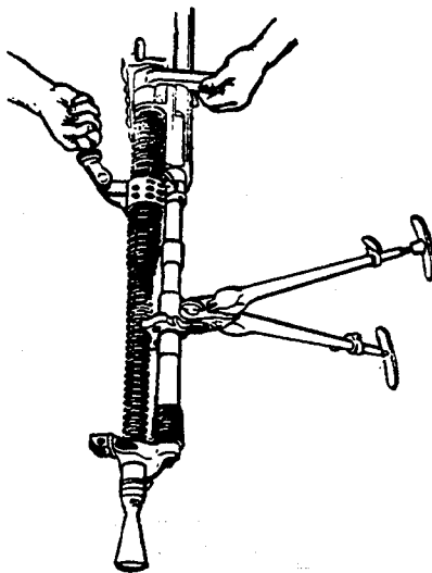
图 2-60 卸下枪管
