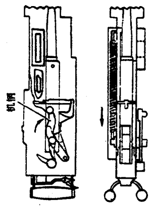
图 2-66 枪机后退示意图
