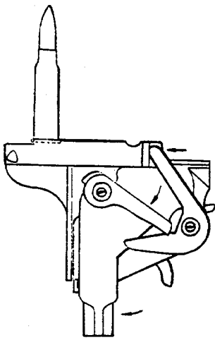
图 2-68 卡上第一发子弹
