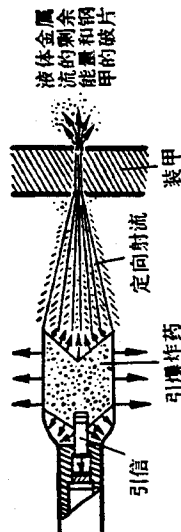
图 6-15 火箭弹破甲示意图
