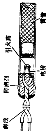
图 3-60 电雷管
